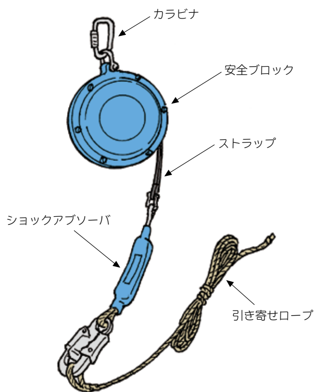
安全ブロック
