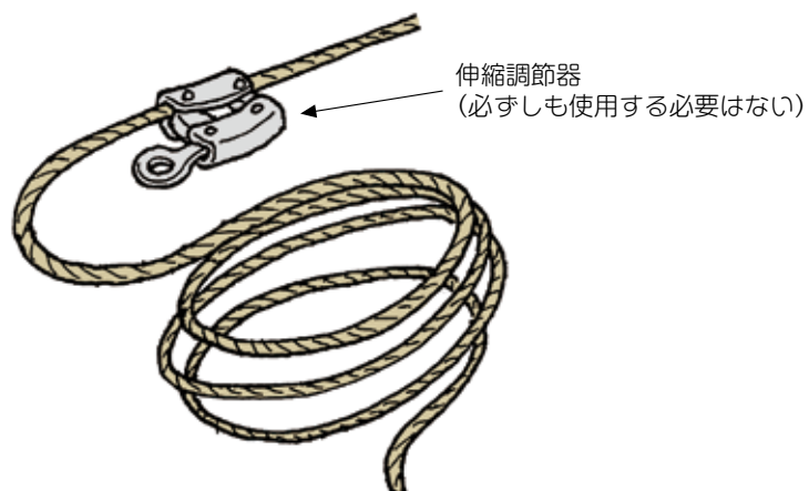
はしご固定ロープ
